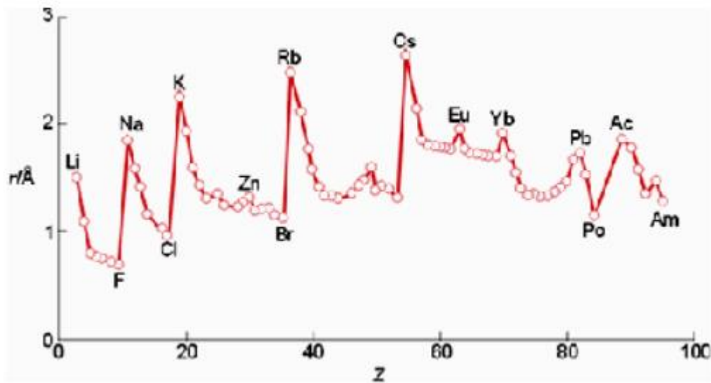
Gráfica 1: Germán Tomás. Variación del radio atómico (Gráfica). Recuperado de http://iesdmjac.educa.aragon.es/departamentos/fq/temasweb/fqdmiral/QUI2BAC/QUI2BAC%20Tema%207%20Estructura%20atomica%20y%20sistema%20periodico/81_radio_atmico.html . Consultado el 31/05/2020
